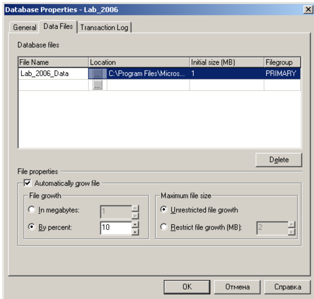
Рис 3.3. Вкладка Data Files
