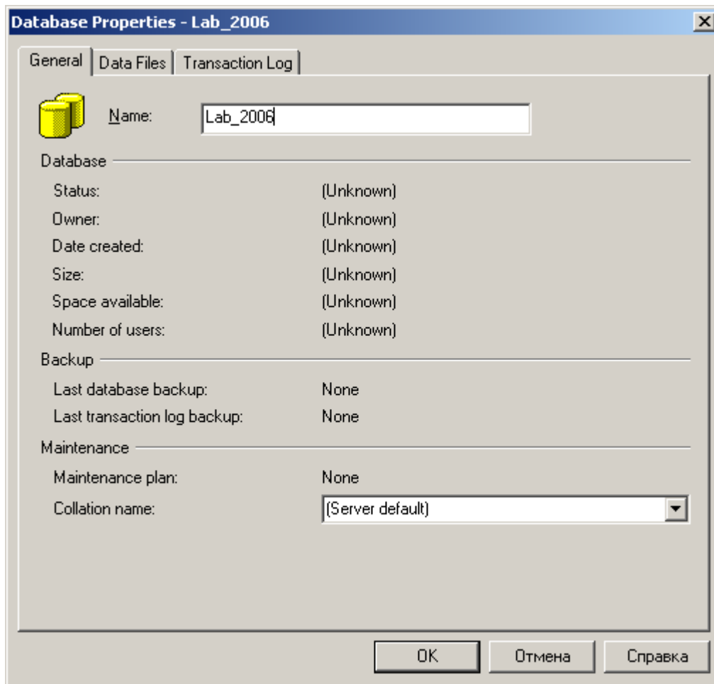
Рис 3.2. Вкладка General
