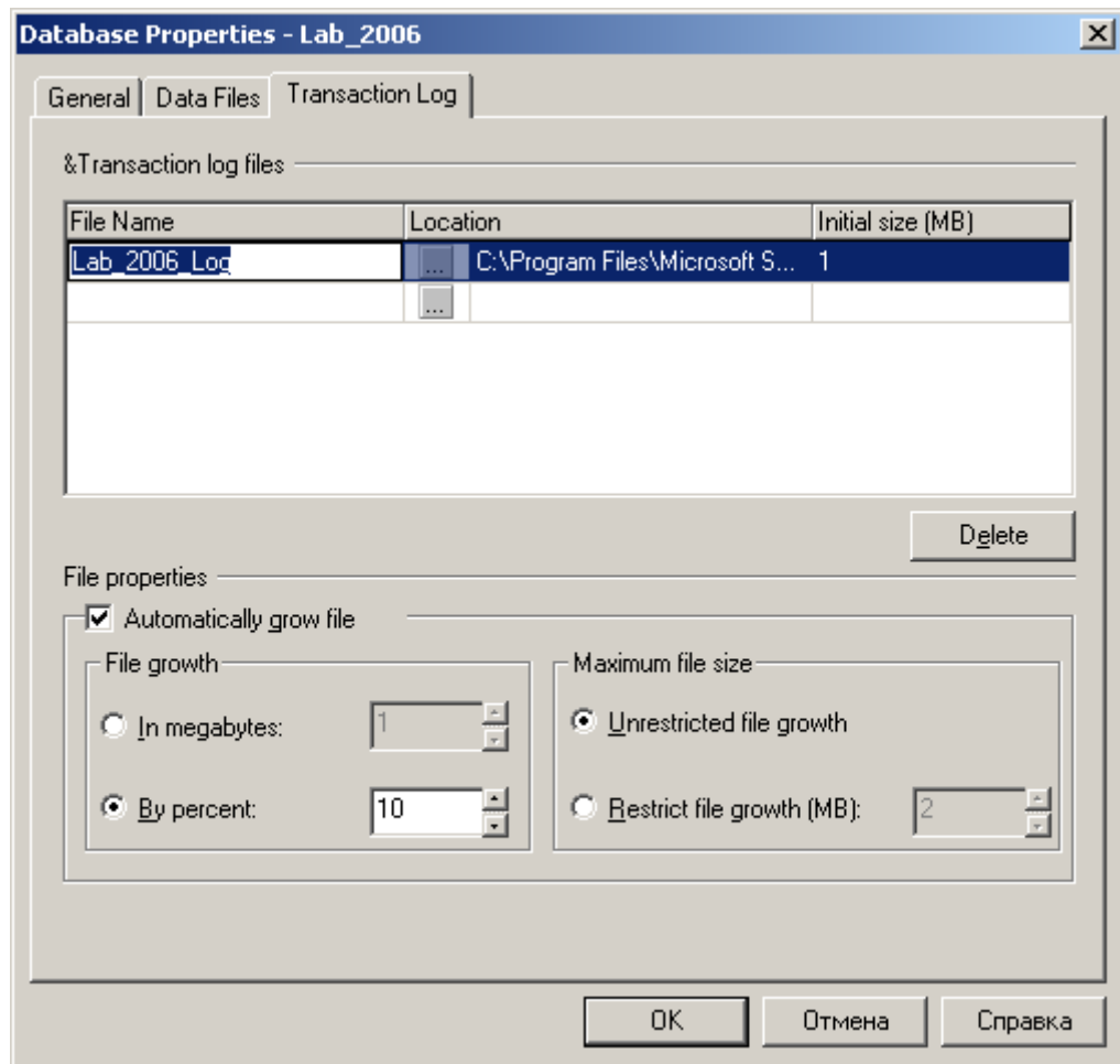
Рис 3.4. Вкладка Transaction_log
