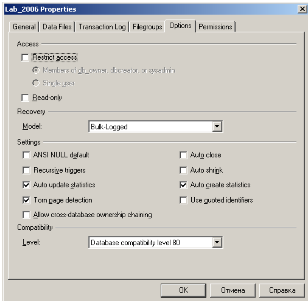
Рис 3.5. Вкладка OPTIONS
