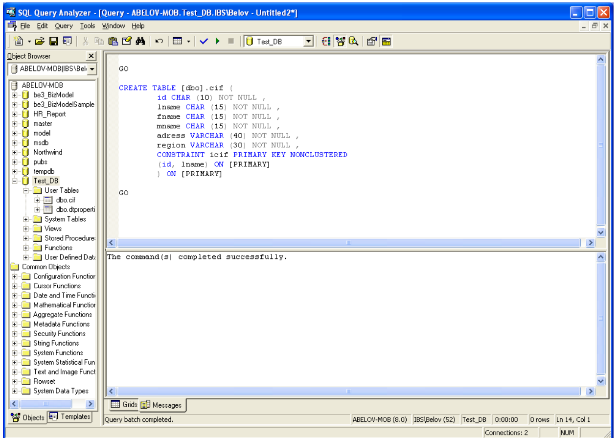
Рис. 3.8. Создание таблицы средствами SQL Query Analyzer
