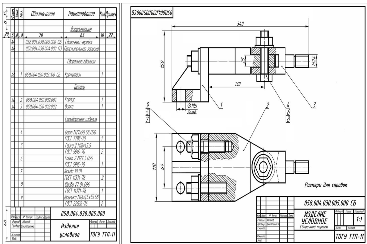
Рисунок 4 – Пример оформления сборочного чертежа.
