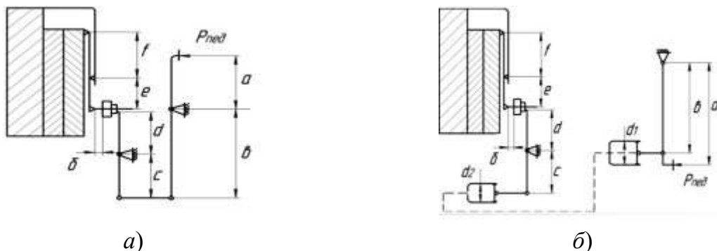
Рисунок 3 - Схемы приводов сцепления: a – механический привод; б – гидравлический привод
