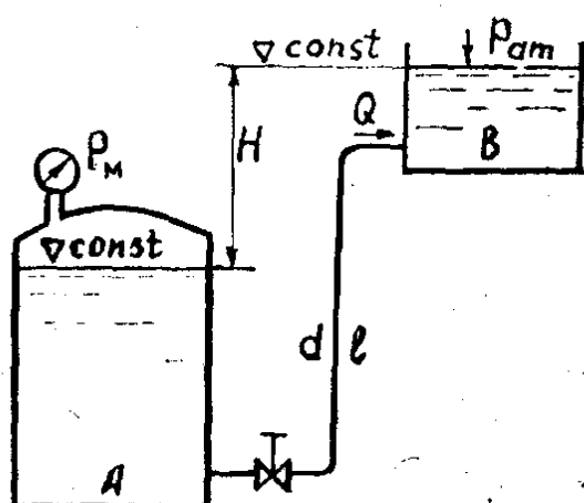
Р и с. 4. Гидравлический расчет коротких трубопроводов
