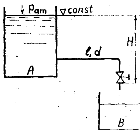
Р и с. 4. Гидравлический расчет коротких трубопроводов
