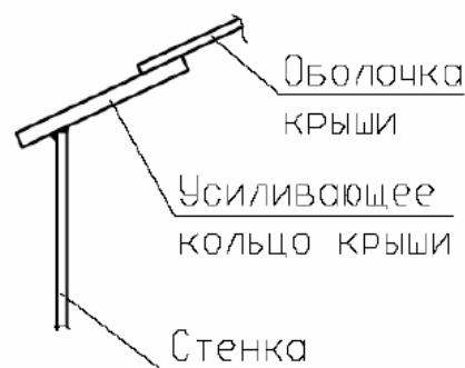
Рисунок 3 - Узел сопряжения самонесущих конических и купольных крыш со стенкой резервуара
