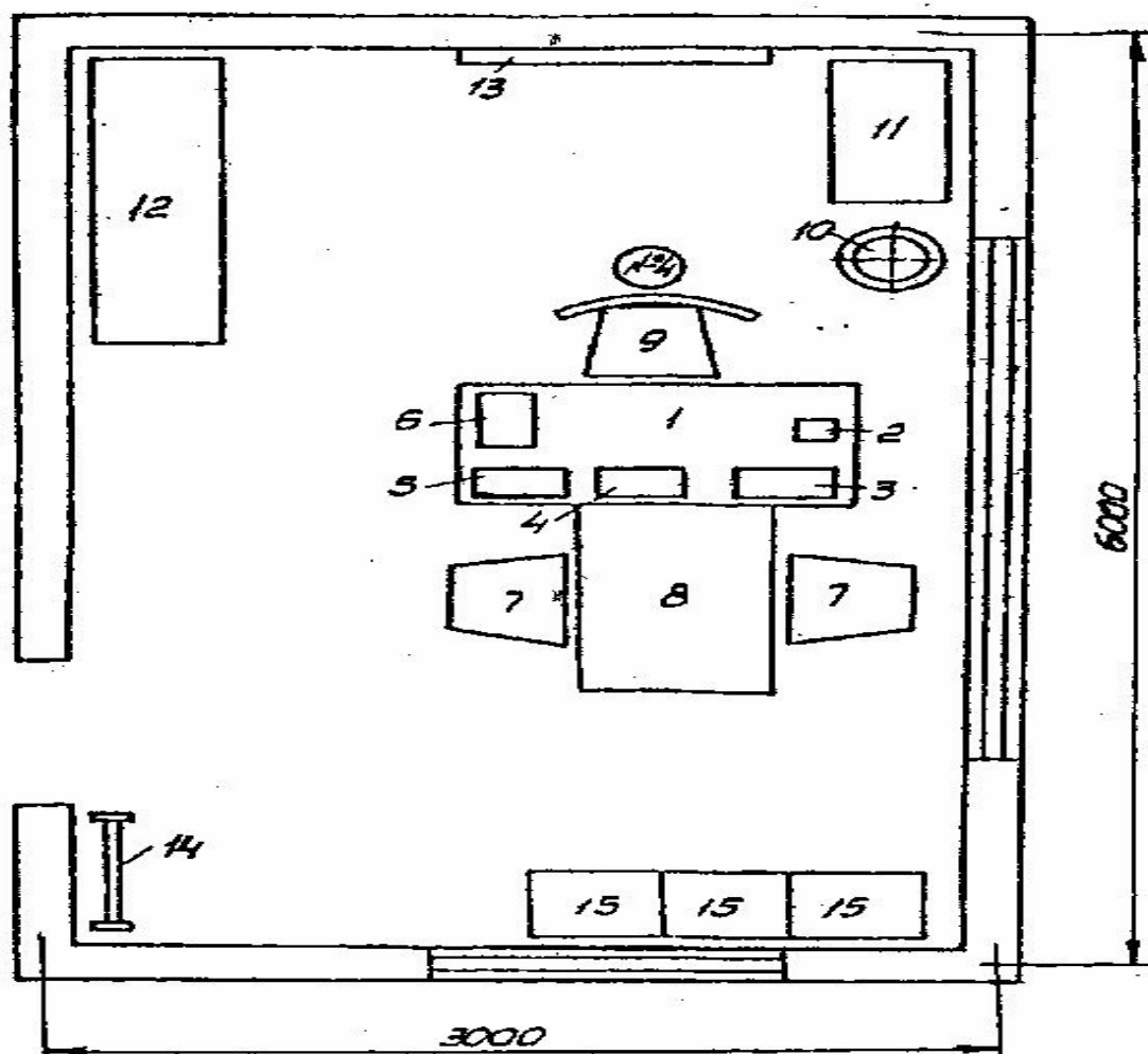
Экспликация оборудования
