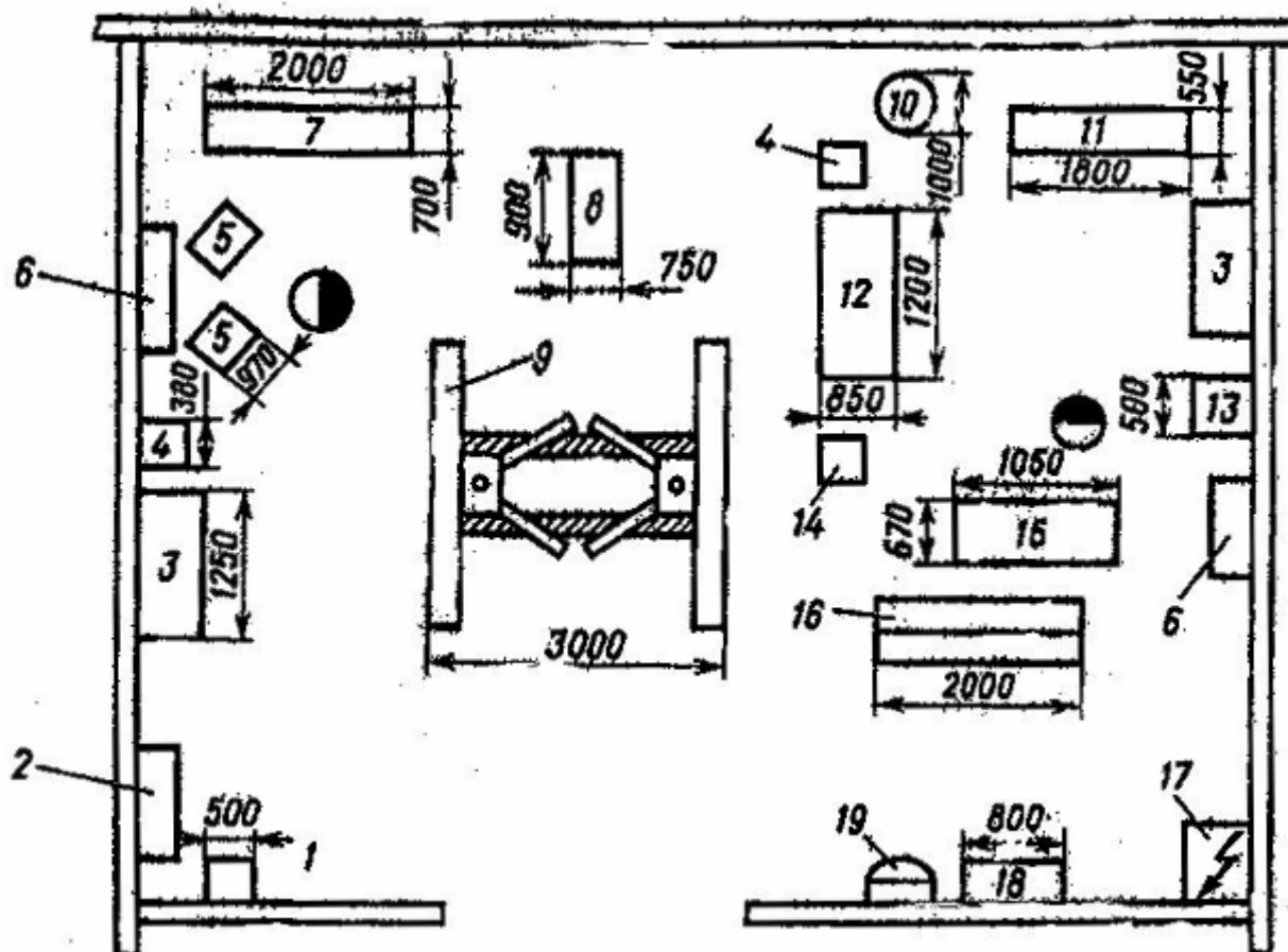
Экспликация оборудования
