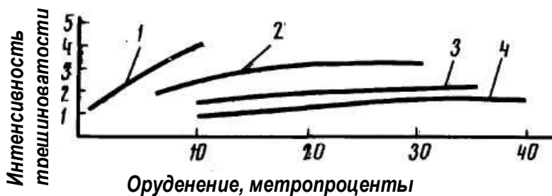
Рис. 3.16. Зависимость интенсивности трещиноватости ( W ) от оруденения ( c ): 1 — залежь «Покро 7а»; 2 — залежь «Кресто — 9»; 3 — залежь «Покро — 7»; 4 — залежь «Кресто — 8».
