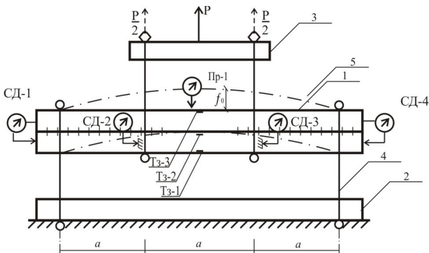
Рис. 5.3. Схема испытательной установки на машине Р-10: 1 – образец составной балки с упругоподатливыми связями; 2 – неподвижная траверса; 3 – подвижная траверса; 4 – тяжи с опорами; 5 – линия изгиба балки
