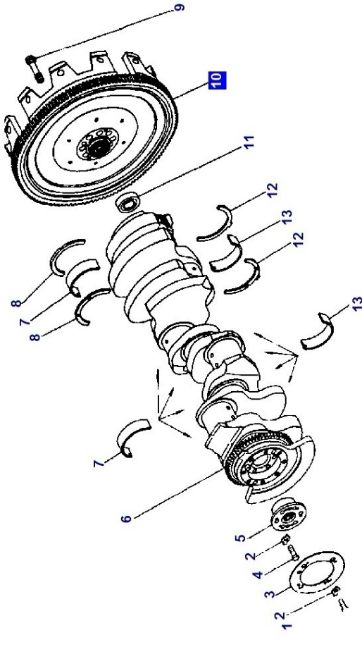
Маховик в сборе
