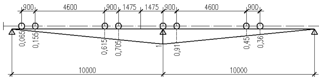
Рис. 3. Линии влияния давления кранов
