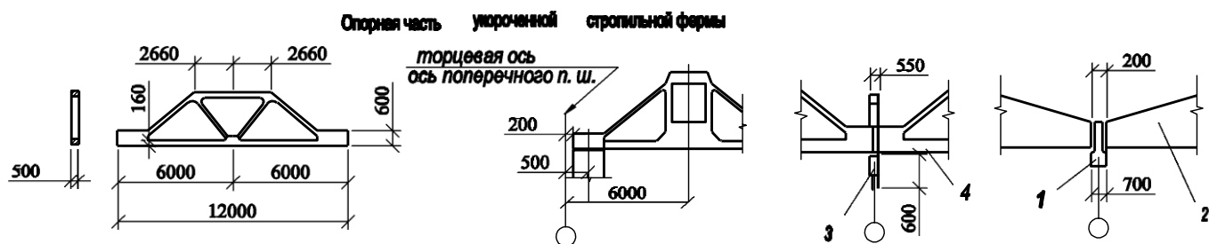
1 - подстропильная балка
