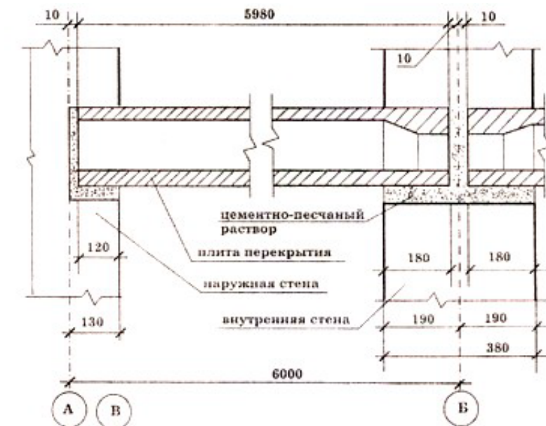
Рис.7.Привязканесущихстен
