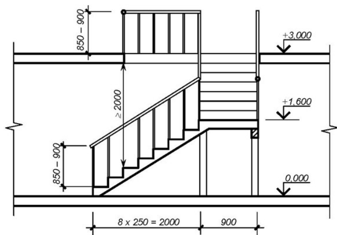
Рис. 6. Схемавнутриквартирнойлестницысповоротомна90°: внижнеммарше8ступенейвысотой200мм,вверхнем—7 ступеней
