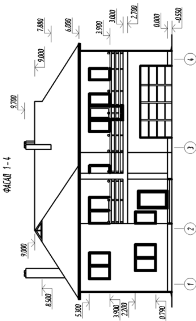
Фасад1-4
