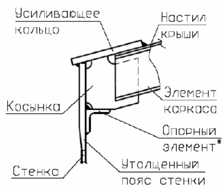
Рисунок 4 - Узел сопряжения каркасных конических и сферических крыш со стенкой резервуара
