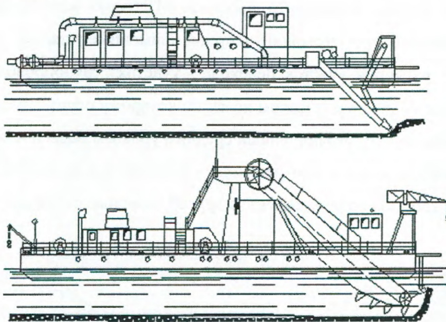
Рис. 1.5 - Землечерпательный снаряд [6]
