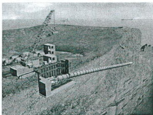
Рис. 1.9 – Метод микротоннелирования [6]
