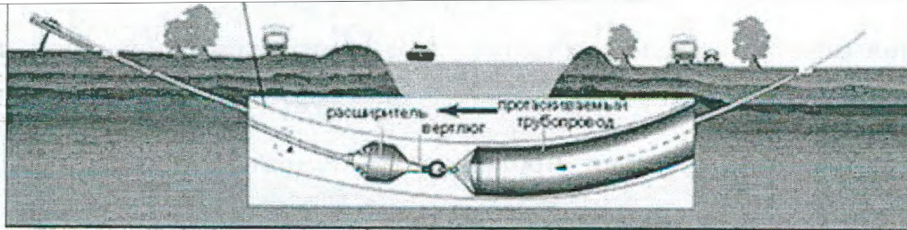
Рис. 1. 6 – Метод прокладки способом наклонно – направленного бурения [6]
