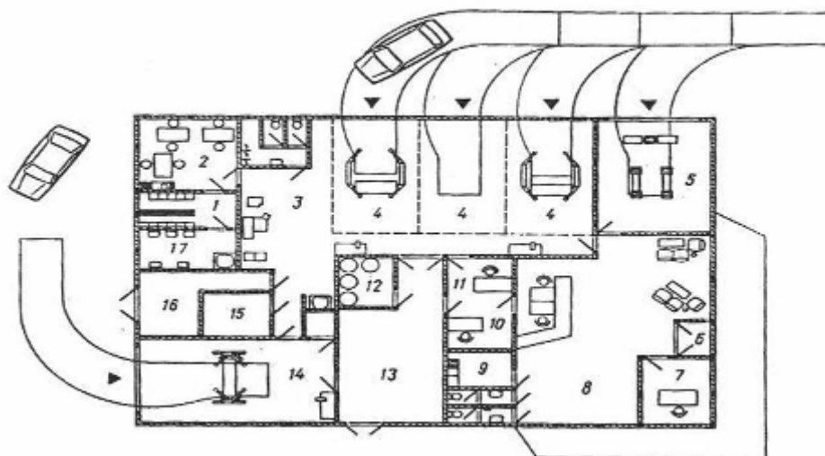
Экспликация помещений
