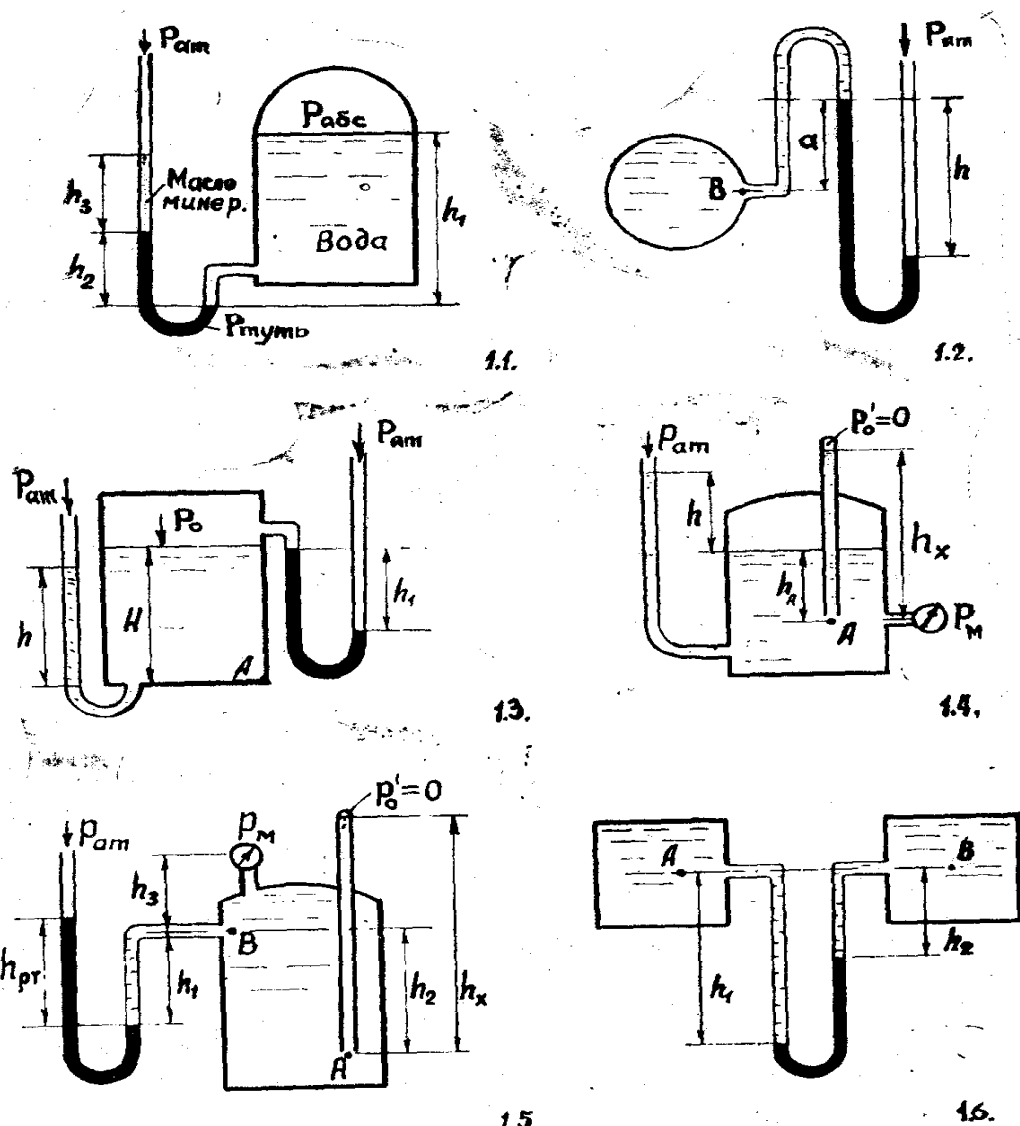
Рис. 1. Гидростатическое давление и его измерение
