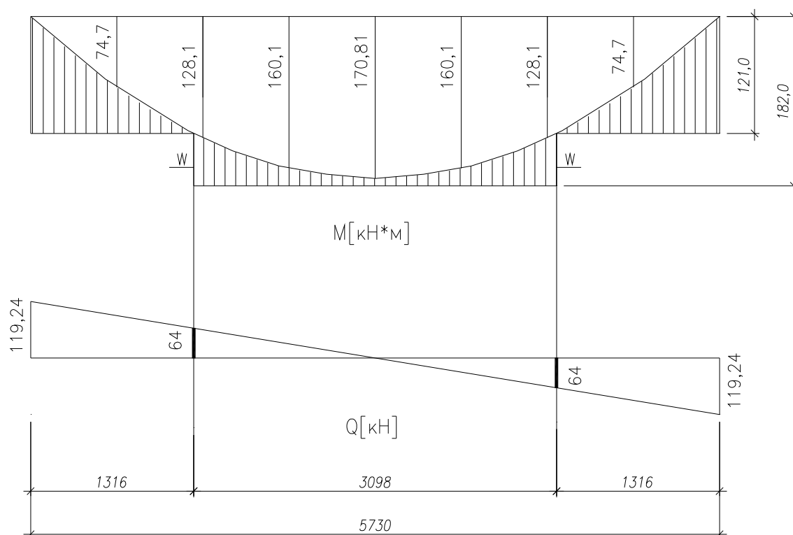
Рис. 10. Эюра материалов
