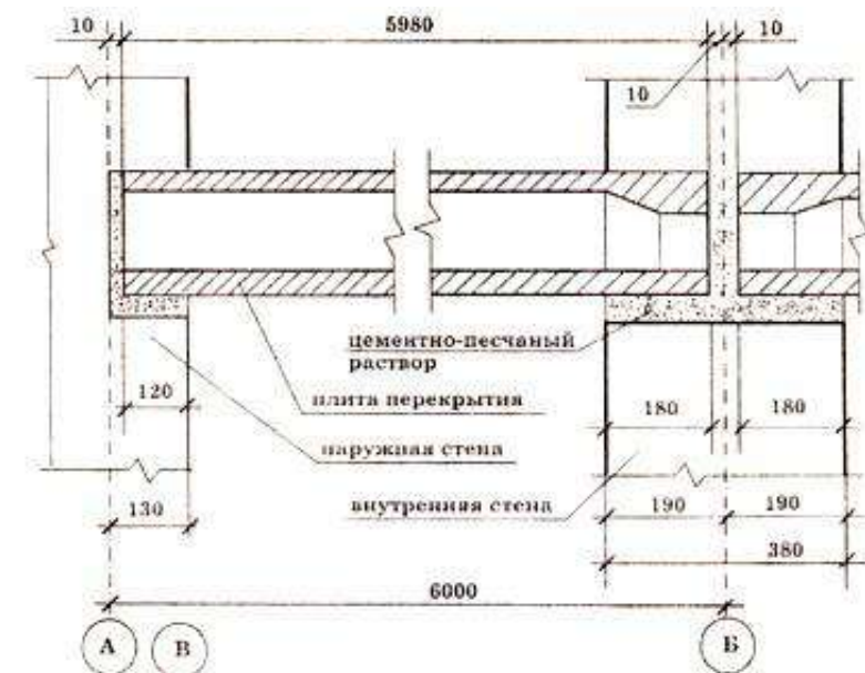
Рис. 7. Привязка несущих стен
