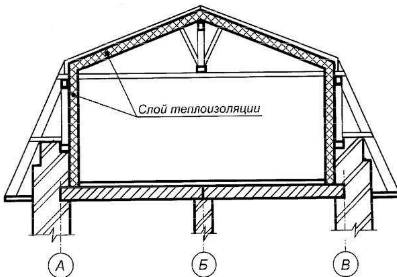
Рис.13.Окончание: б-приотапливаемой(жилой)мансарде
