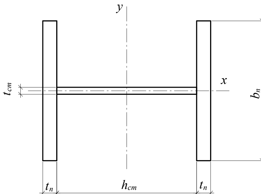
Рис. 13. Поперечное сечение колонны
