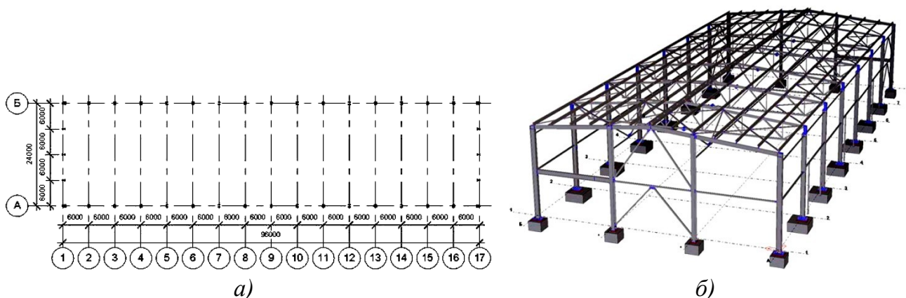
Рисунок 6.1 – Компоновка здания производственного корпуса АТП
