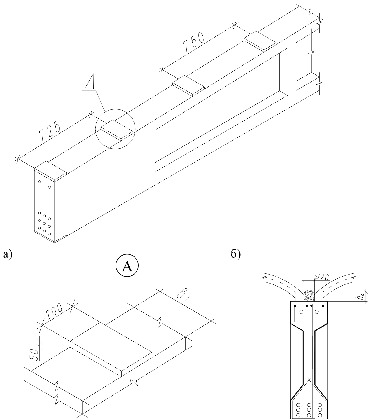
Рис. 15. Бортовой элемент а) Бетонные шипы бортового элемента. б) Опираение панелей на бортовой элемент.
