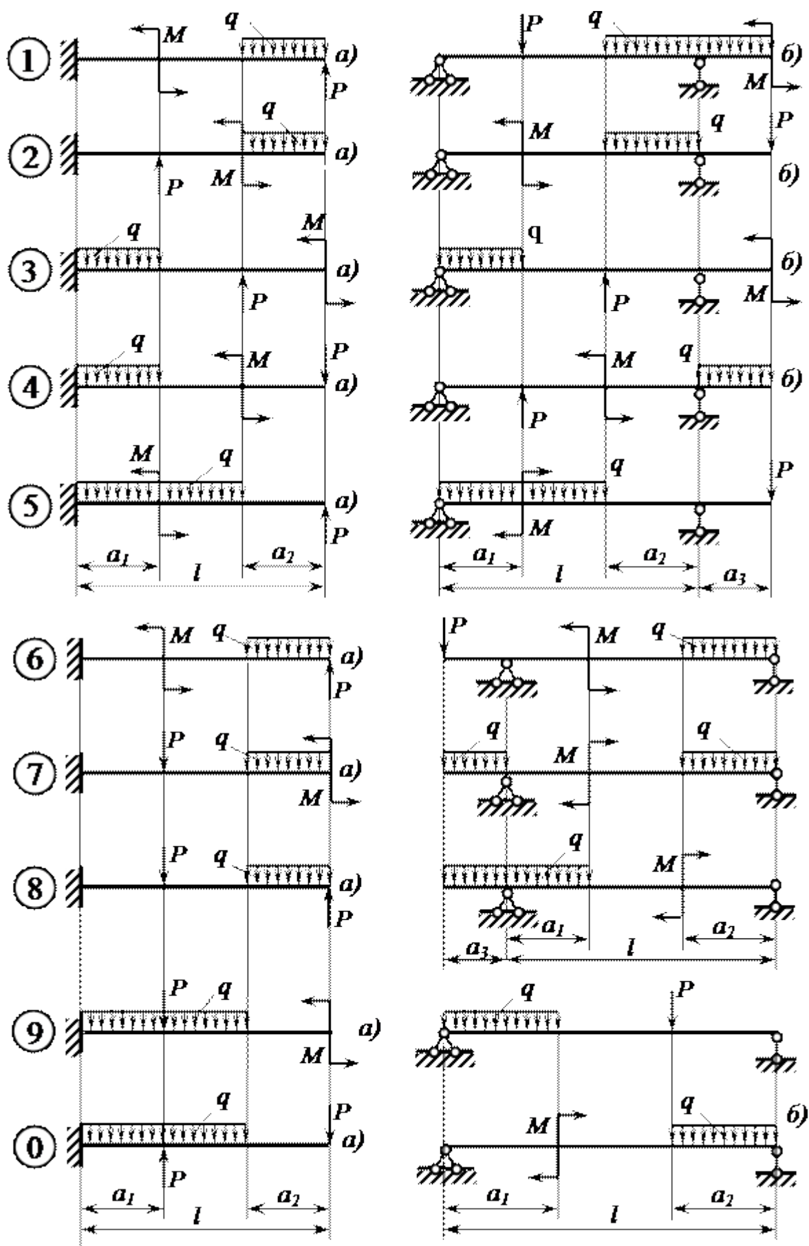
Рис.7 Расчетные схемы
