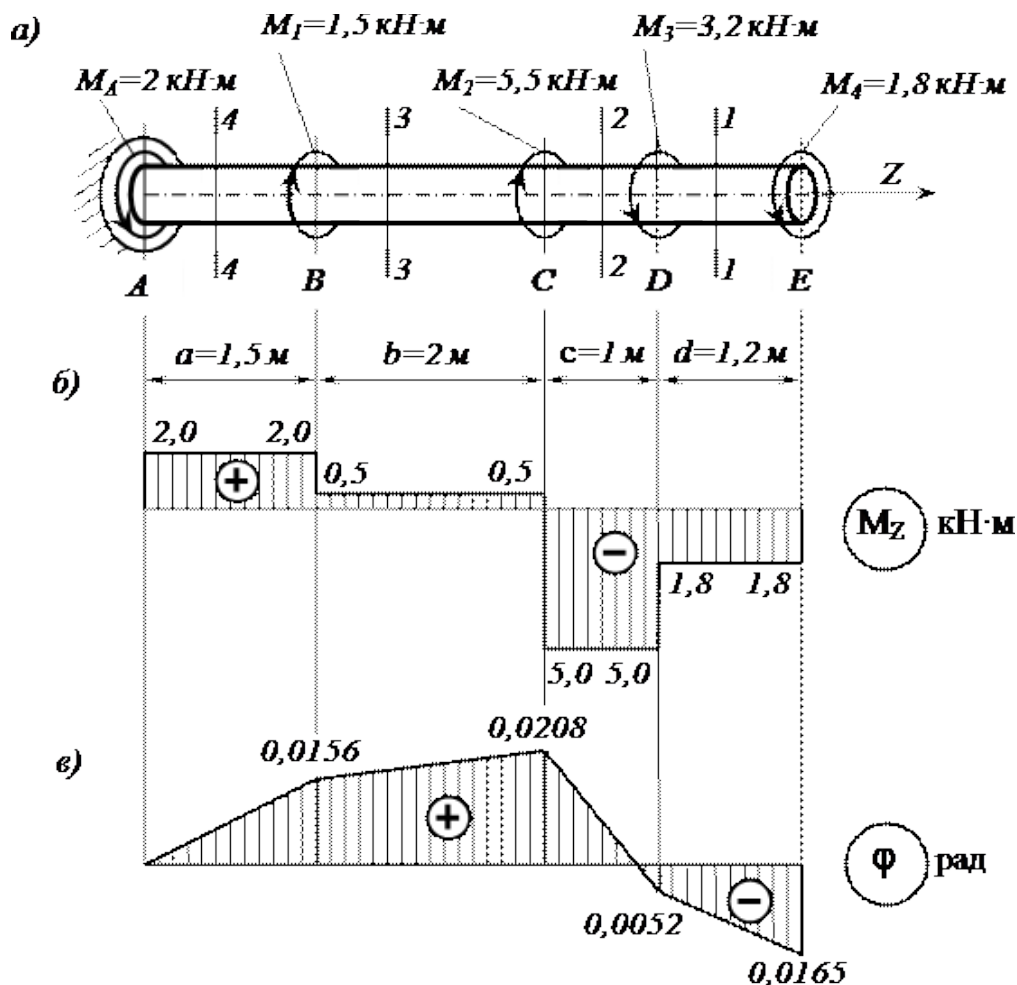
Рис. 5 Расчетная схема
