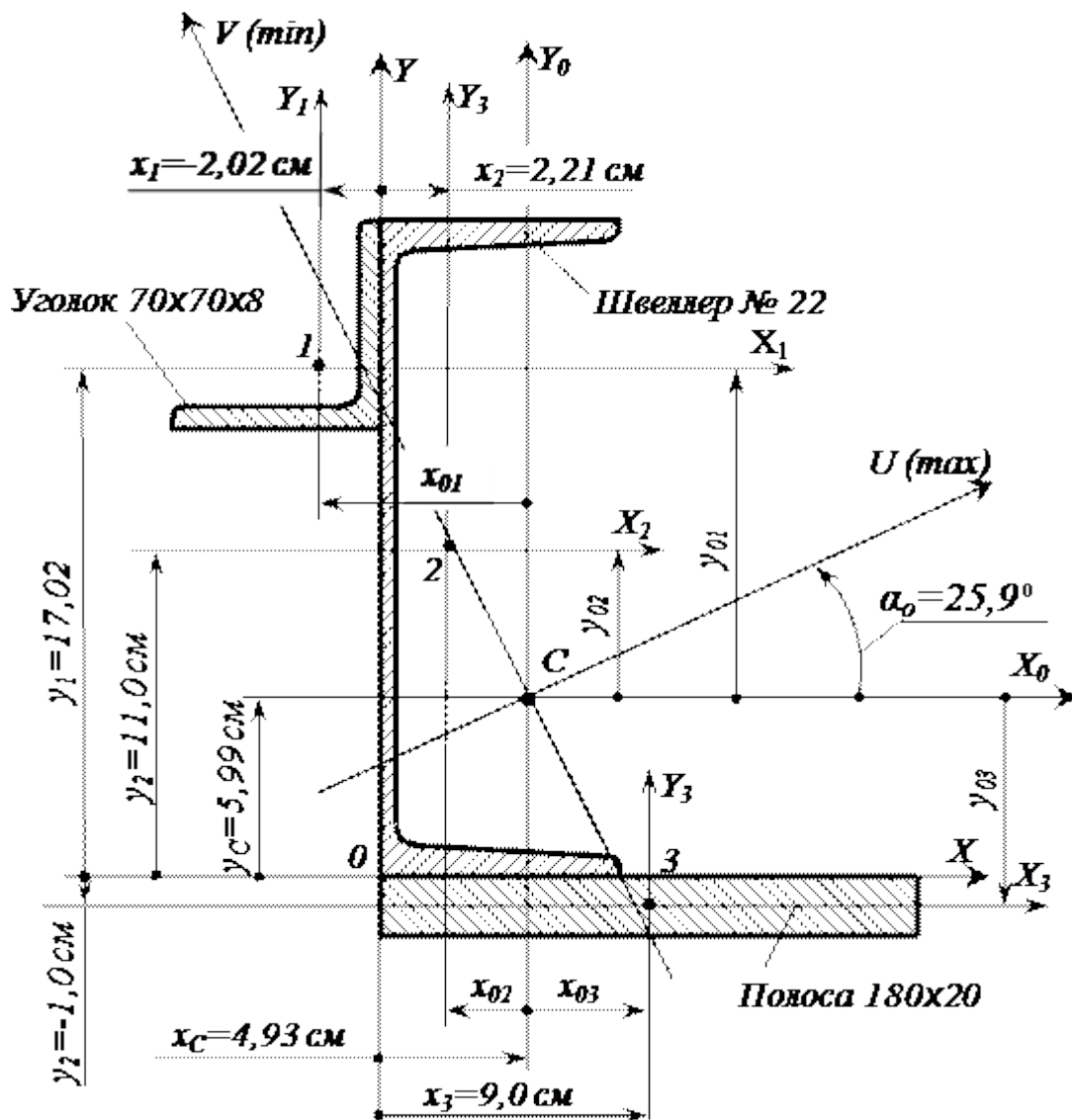
Рис. 8 Расчетная схема
