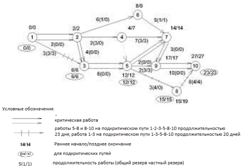
Рис.7. Сетевой график, рассчитанный методом дроби с указанием критического и подкритического пути
