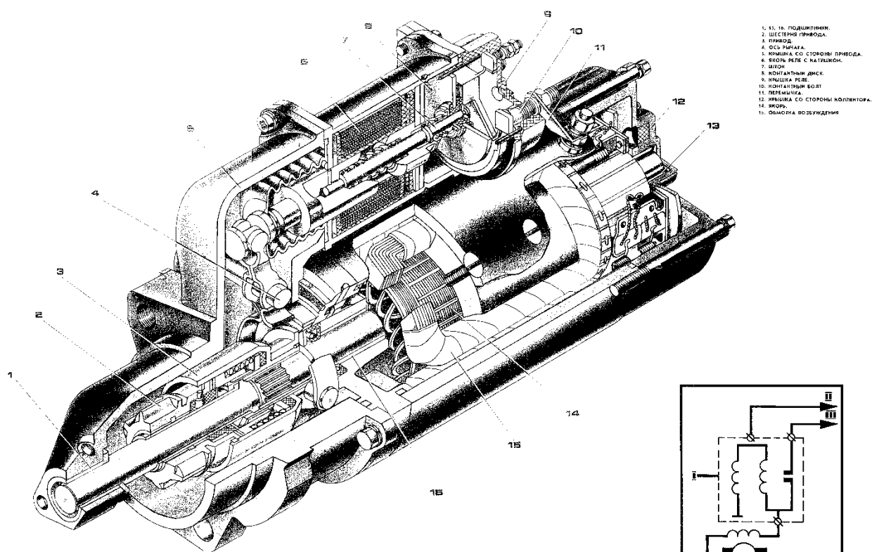
I. ТЯГОВОЕ РЕЛЕ СТАРТЕРА. II. И ВЫКЛЮЧАТЕЛЬНОЕ ПРИБОРОМ И СТАРТЕРА. III. И АККУМУЛЯТОРНАЯ БАТАРЕЯ.
