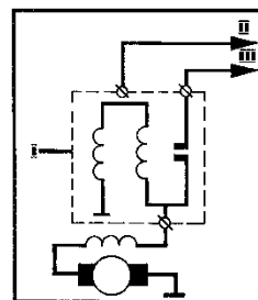
I. ТЯГОВОЕ РЕЛЕ СТАРТЕРА. II. И ВЫКЛЮЧАТЕЛЬНОЕ ПРИБОРОМ И СТАРТЕРА. III. И АККУМУЛЯТОРНАЯ БАТАРЕЯ.
