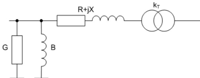
Рисунок - Г-образная схема замещения
