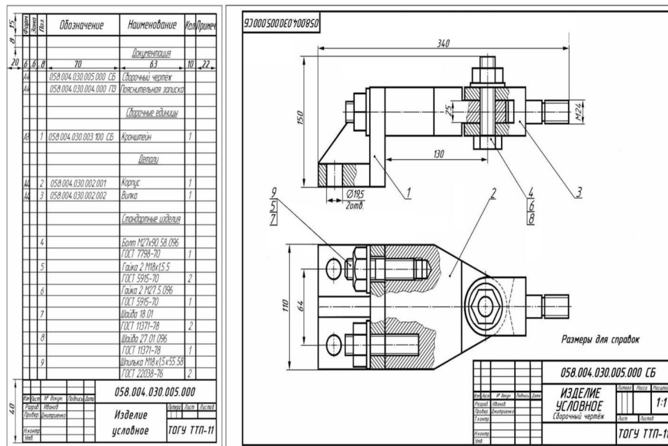
Пример оформления сборочного чертежа
