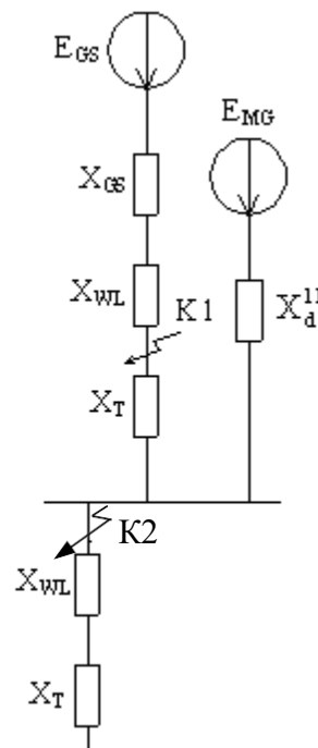
Рисунок 15– Схема замещения
