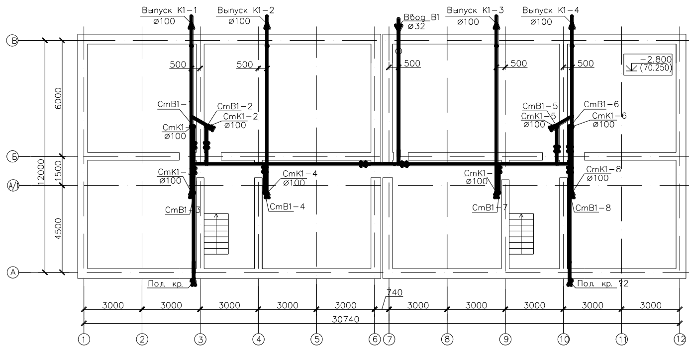
ПЛАН ПОДВАЛА
