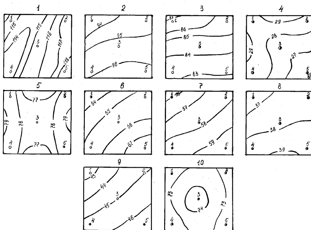
Рис. 9. Топографические планы строительных площадок, М 1:10000
