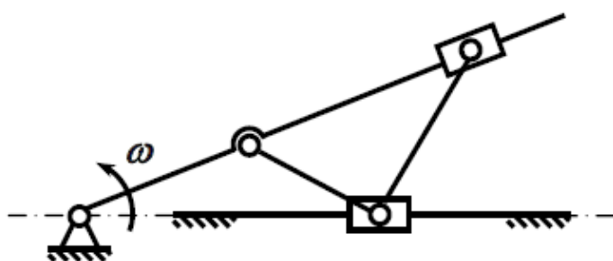
Рис.1.1. Механизм трисектора
