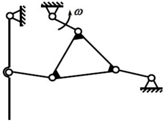
Рис.1.12. Механизм дробилки
