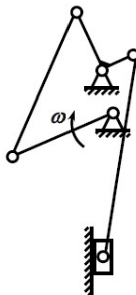
Рис.1.5. Механизм вытяжного прессы
