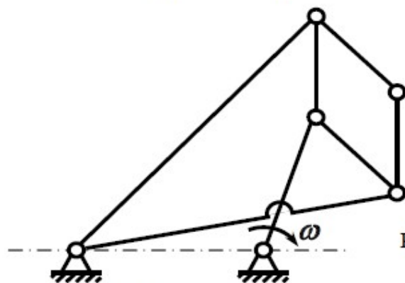
Рис.1.6. Механизм Липкина
