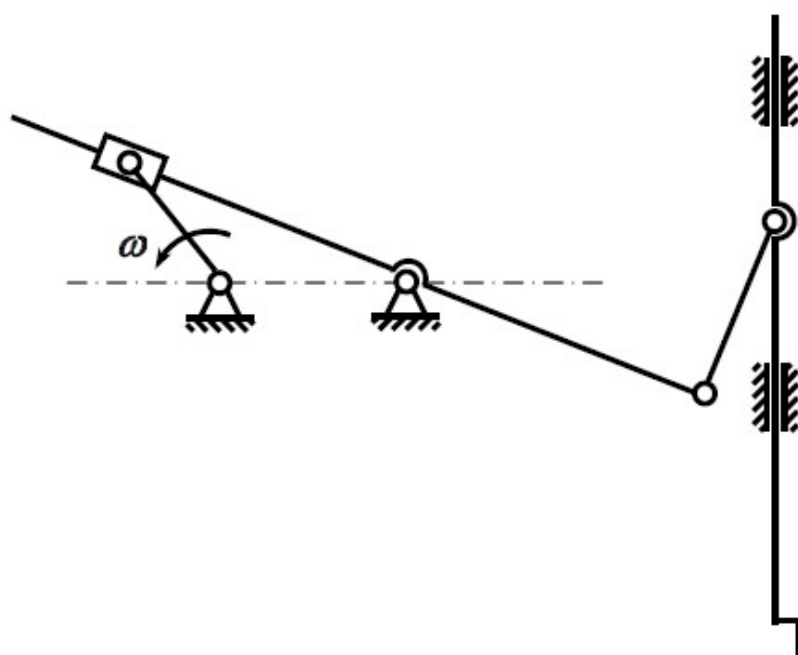
Рис.1.18. Механизм перемещения долбьяка
