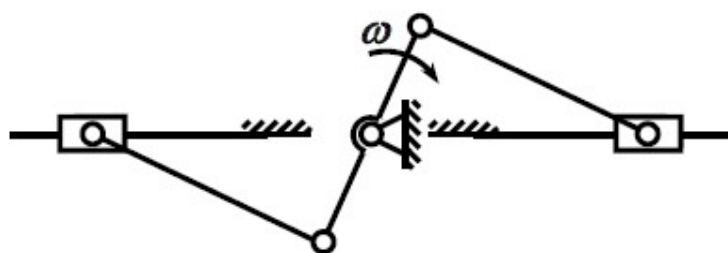
Рис.1.4. Механизм двухцилиндрового опозитного четырехтактного двигателя внутреннего сгорания
