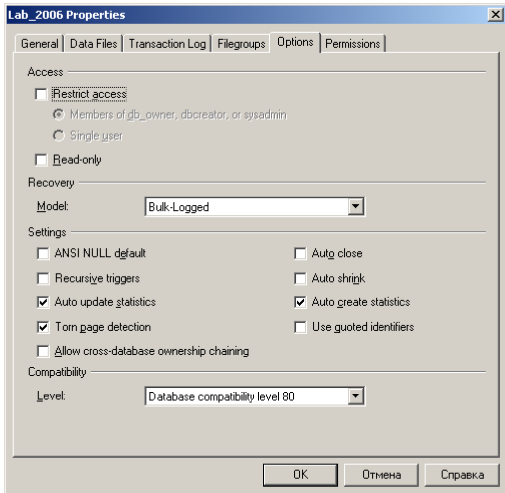
Рис 3.5. Вкладка OPTIONS
