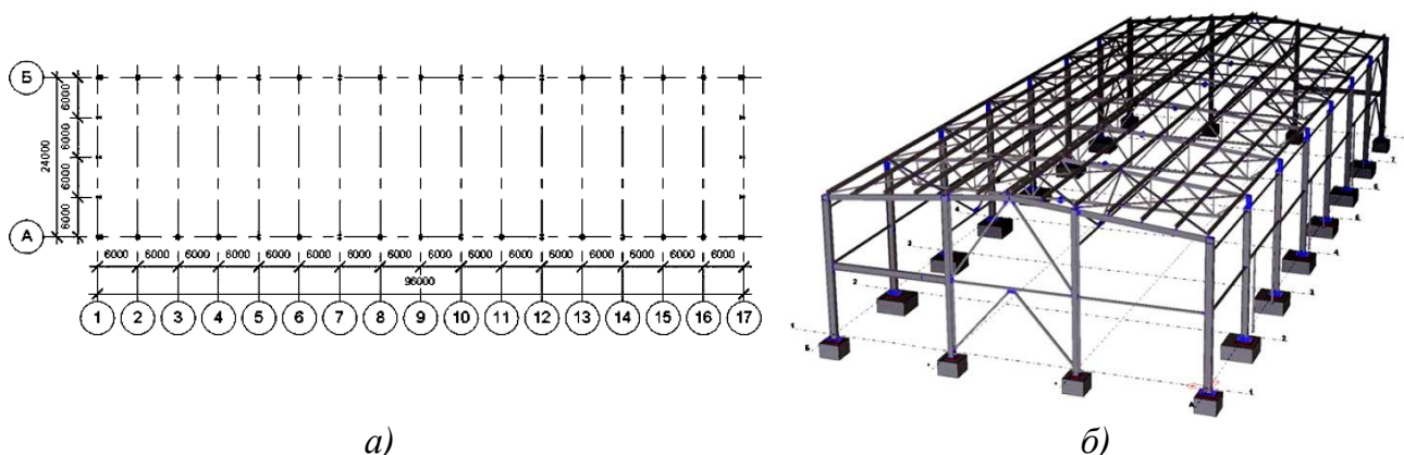
Рисунок 6.1 – Компоновка здания производственного корпуса АТП а) конструктивная схема; б) 3D модель
