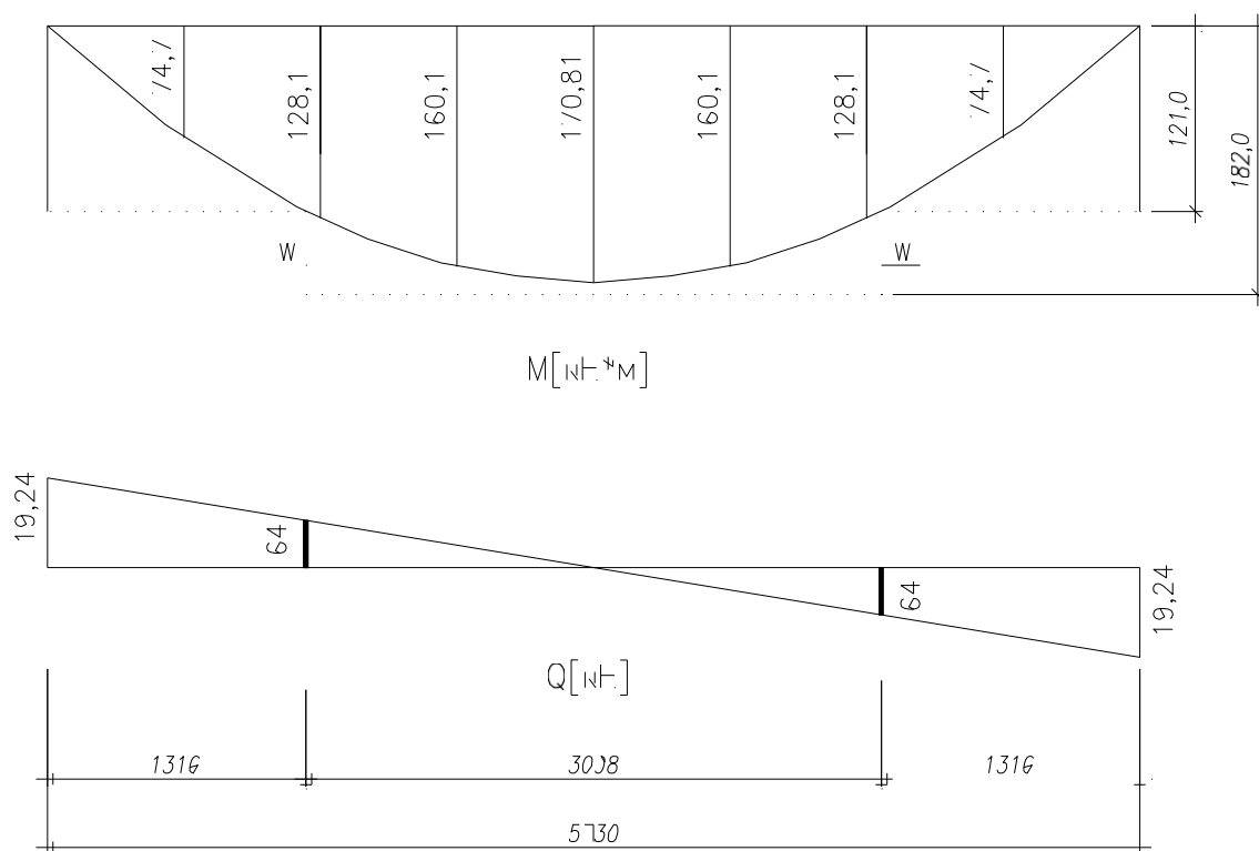
Рис. 10. Эпюра материалов
