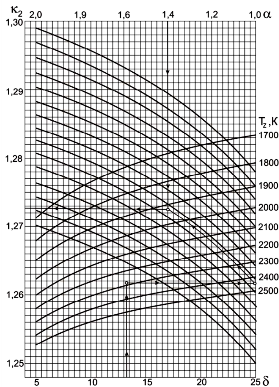
Рисунок 1.2 - Номограмма для определения показателя адиабаты расширения K_2 для дизеля
