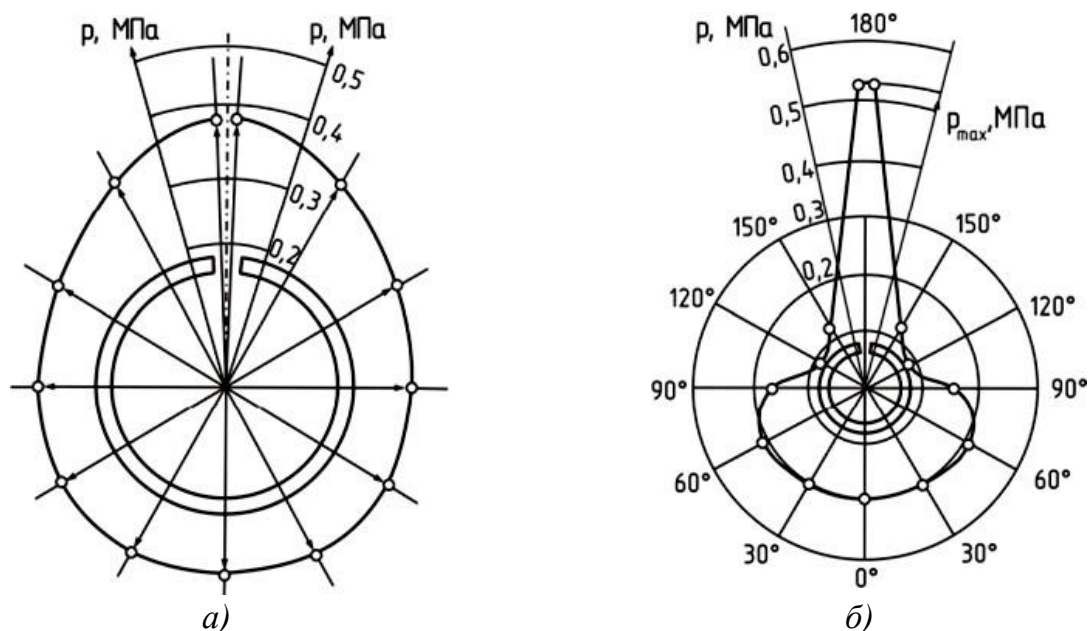
Рисунок 5.2. - Эпюры сил давления кольца на стенку цилиндра: а) – грушевидная эпюра давлений (для бензинового двигателя); б) – каплевидная эпюра давлений (для дизеля)
