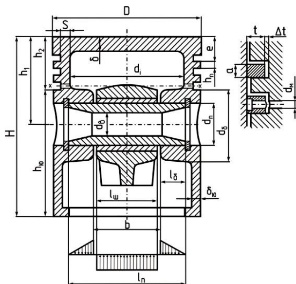
Рисунок 5.1 - Схема поршня
