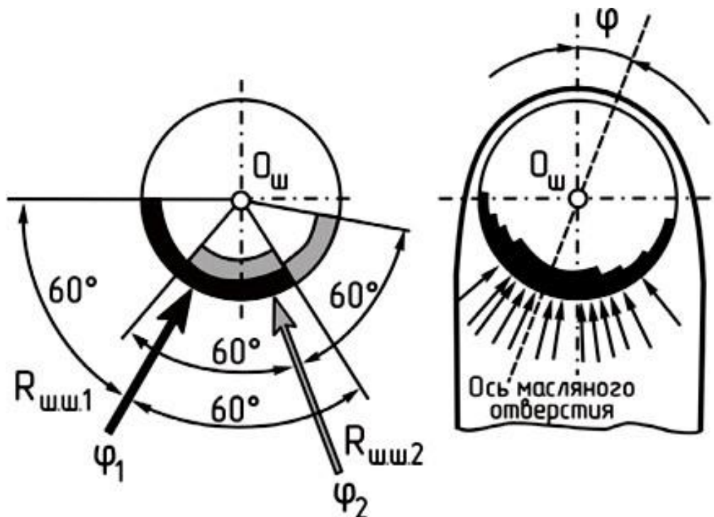
Рисунок 2.5 – Схема построения диаграммы износа шатунной шейки
