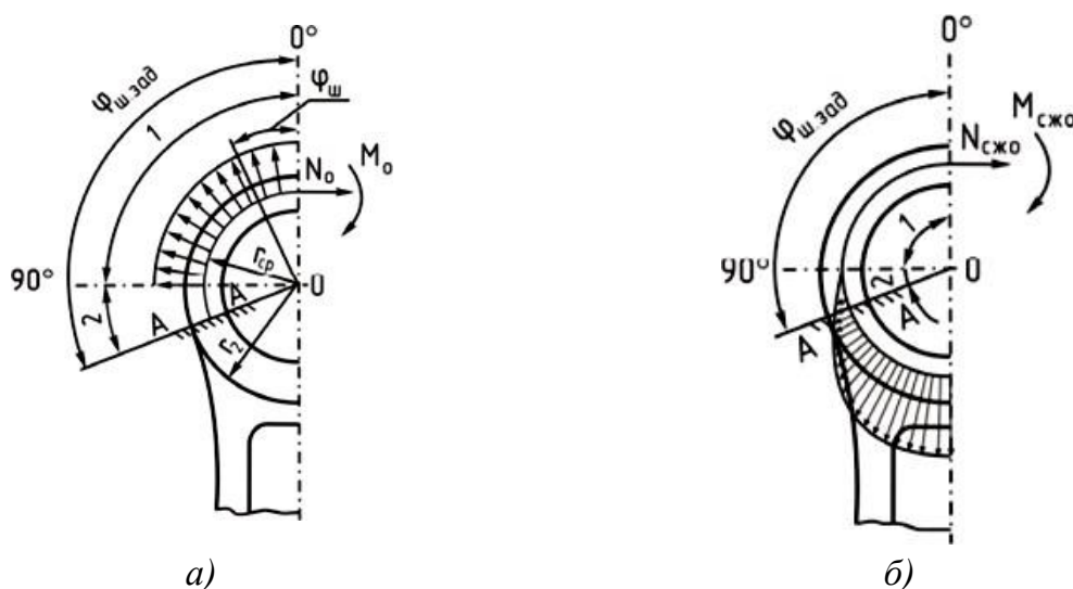
Рисунок 5.4 - Схема распределения нагрузок на поршневую головку шатуна: а) при растяжении; б) при сжатии
