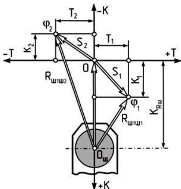
Рисунок 2.3 – Схема построения полярной диаграммы нагрузки на шатунную шейку
