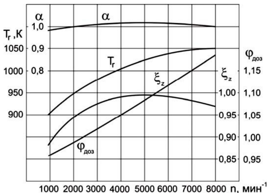
Рисунок 1.4 - Исходные параметры для теплового расчета двигателя с распределенным впрыском топлива
