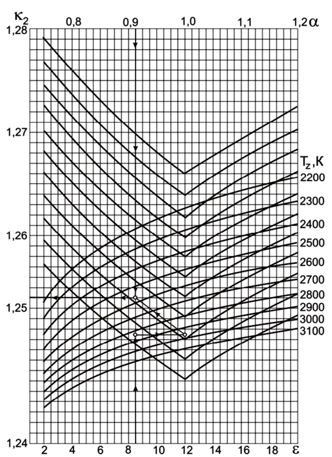
Рисунок 1.3 - Номограмма для определения показателя адиабаты расширения K_2 для бензинового двигателя
