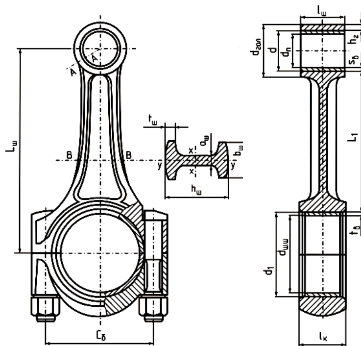
Рисунок 5.3 - Расчетная схема шатунной группы
