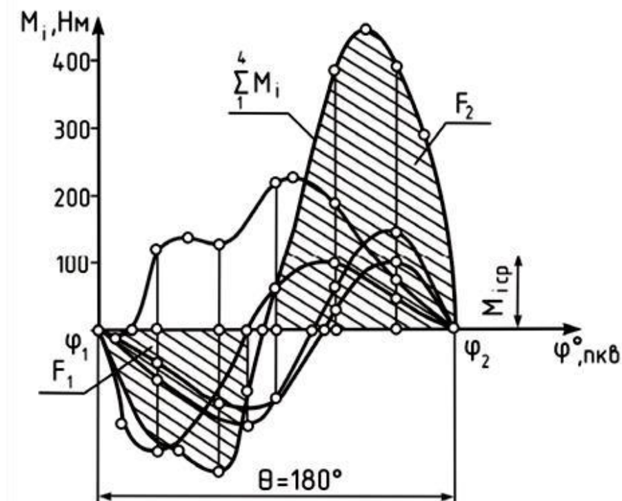
Рисунок 2.6 – Схема построения кривой суммарного крутящего момента
