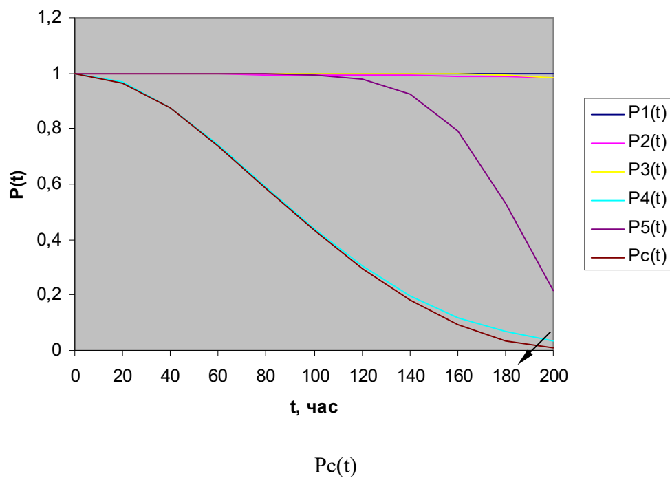
Рис. 1 – Вероятность безотказной работы элементов и системы
