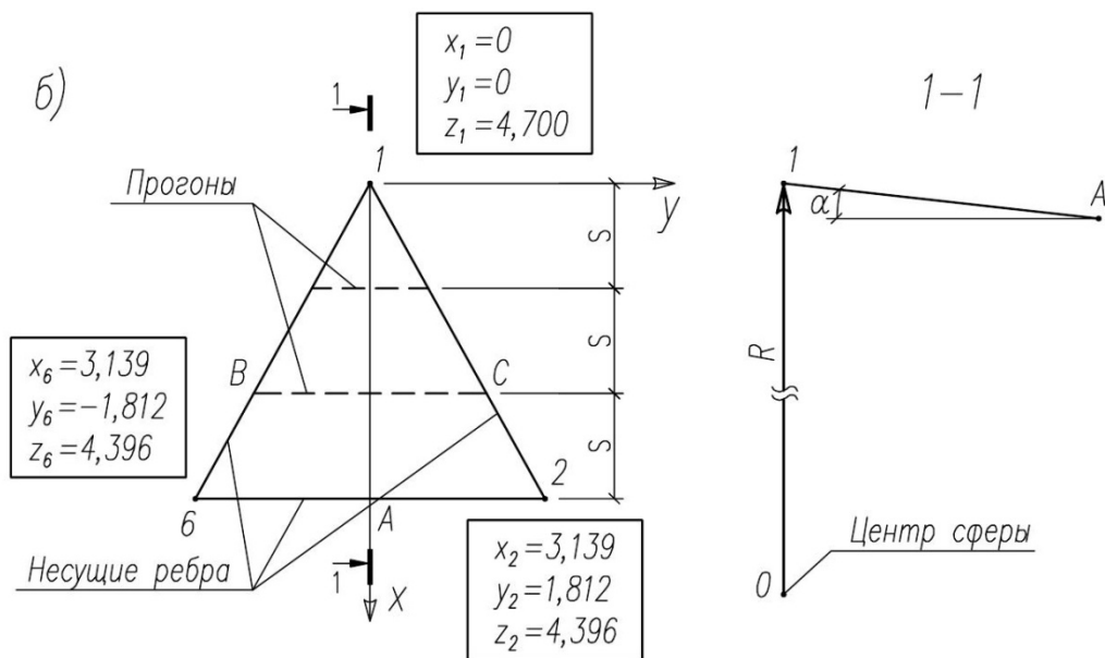
Рис.3. К расчету элементов купола:
