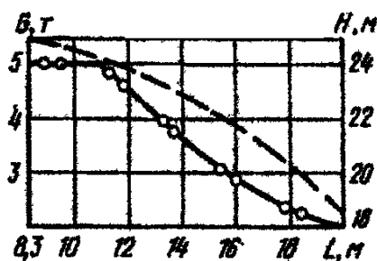
Рис. 4. Слева График грузоподъемности МКГ-25 основной подъем стрела 22,5 м Рис. 5. Справа График грузоподъемности МКГ-25 вспомогательный подъем: стрела 22,5 м, гусёк 5 м
