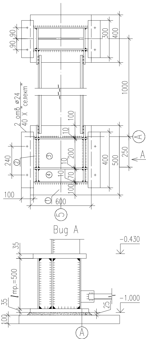
Рис. 8. База колонны
