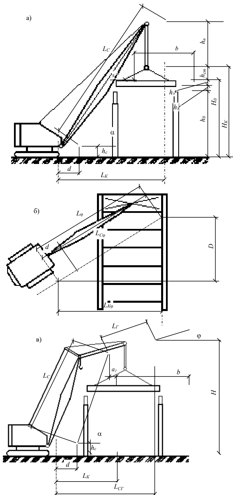
Рис. 3. Расчетные схемы к определению параметрических характеристик(технических параметров): а – стрелового крана без гуська; б – то же, с поворотом в плане; в –стреловогокранагуськом
