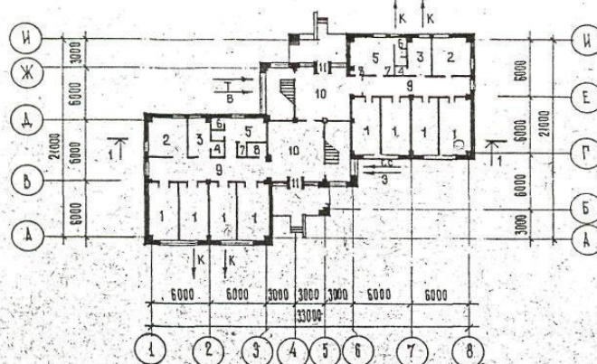
ПЛАН 2 ЭТАЖА
