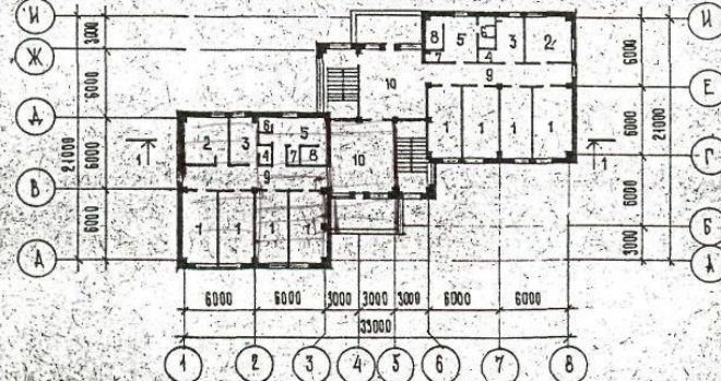
ПЛАН 2 ЭТАЖА
