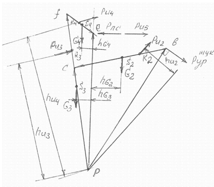
Рис. 5 Рычаг Жуковского
