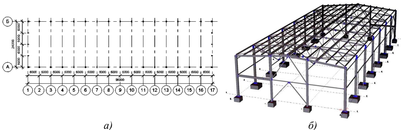
Рисунок 6.1 – Компоновка здания производственного корпуса АТП а) конструктивная схема; б) 3D модель
