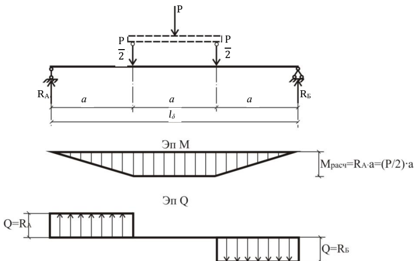
Рис. 4.2. Расчетная схема образца балки и эпюры M и Q
