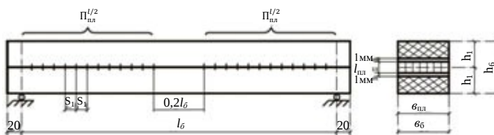
Рис. 5.1. Балка составного сечения с упругоподатливыми связями
