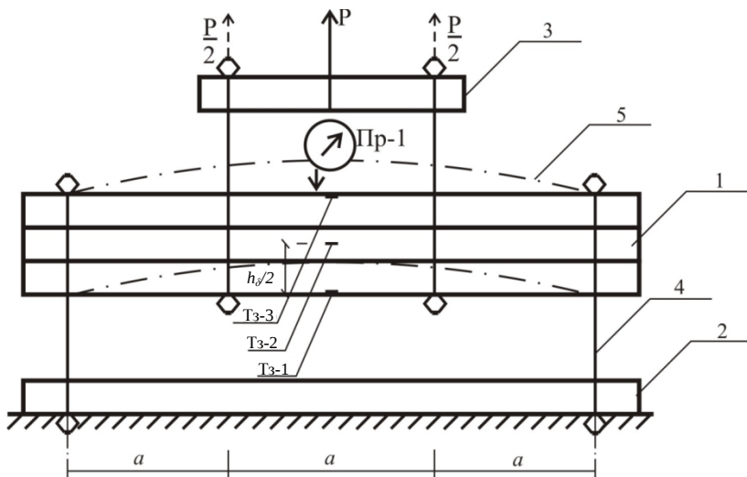
Рис. 3.3. Схема испытательной установки на машине Р-10: 1 – образец клеодоцной балки; 2 – неподвижная траверса; 3 – подвижная траверса; 4 – тяжи с опорами; 5 – линия изгиба балки
