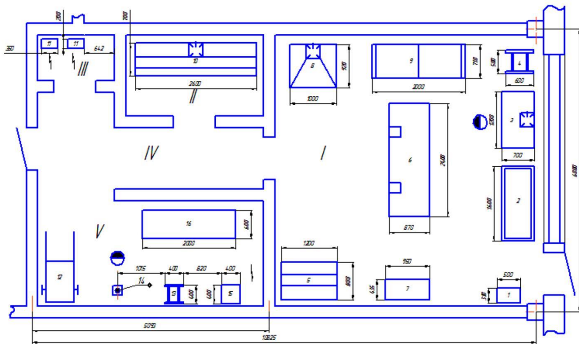
Рисунок 5 – Аккумуляторный участок
