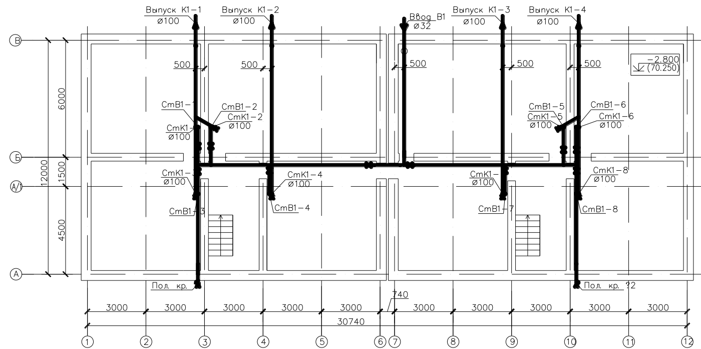
ПЛАН ПОДВАЛА
