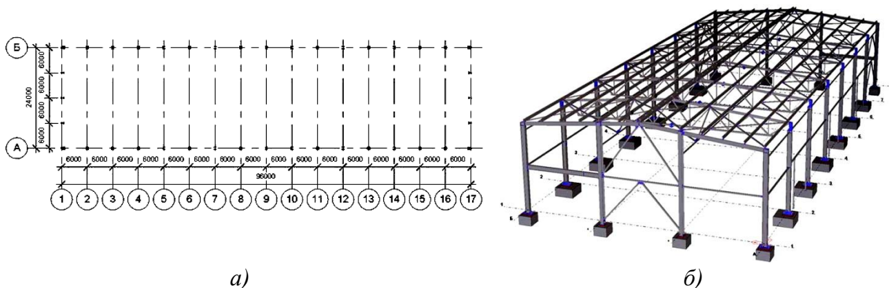
Рисунок 6.1 – Компонка здания производственного корпуса АТП
