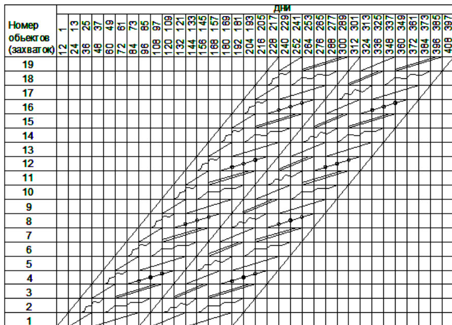
Рис. 6. Циклограмма поточного строительства девятиэтажных жилых домов: I – земляные работы, II – возведение подземной части здания; III – возведение надземной части здания и выполнение I этапа сантехнических и электромонтажных работ; IV – устройство кровли; V – внутренние плотничные работы, затирка стен и потолков, подготовка под полы; VI – отделочные работы, устройство чистых полов, II этап сантехнических и электромонтажных работ; VII – наружное благоустройство.
