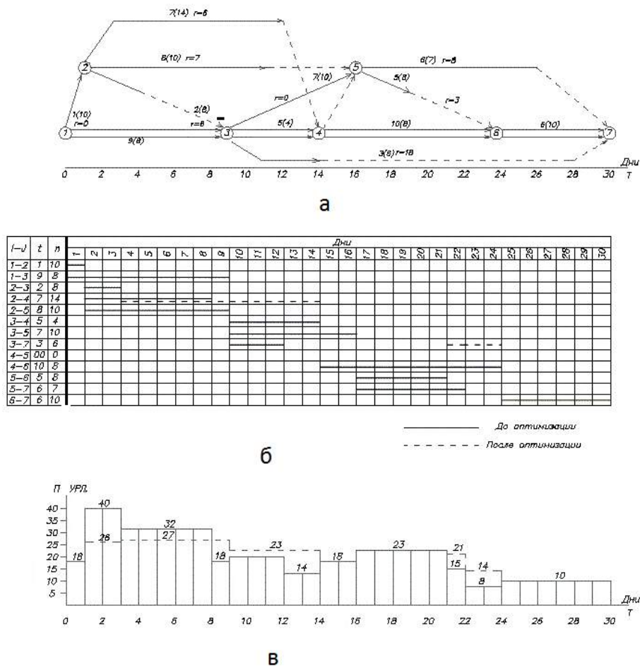
Рис. 13. Оптимизация сетевого графика по рабочим: а – график в масштабе времени до оптимизации; б – линейная диаграмма сетевого графика до и после оптимизации; в – график движения рабочих до и после оптимизации.
