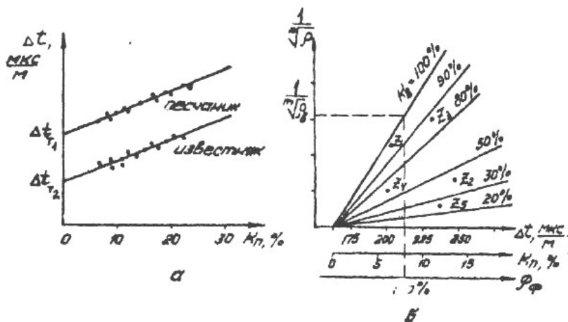
Рис. 3.20. Определение интервального времени \Delta t , соответствующего коэффициенту пористости K_{П} (а); палетка для интерпретации результатов большого объема измерений (б).
