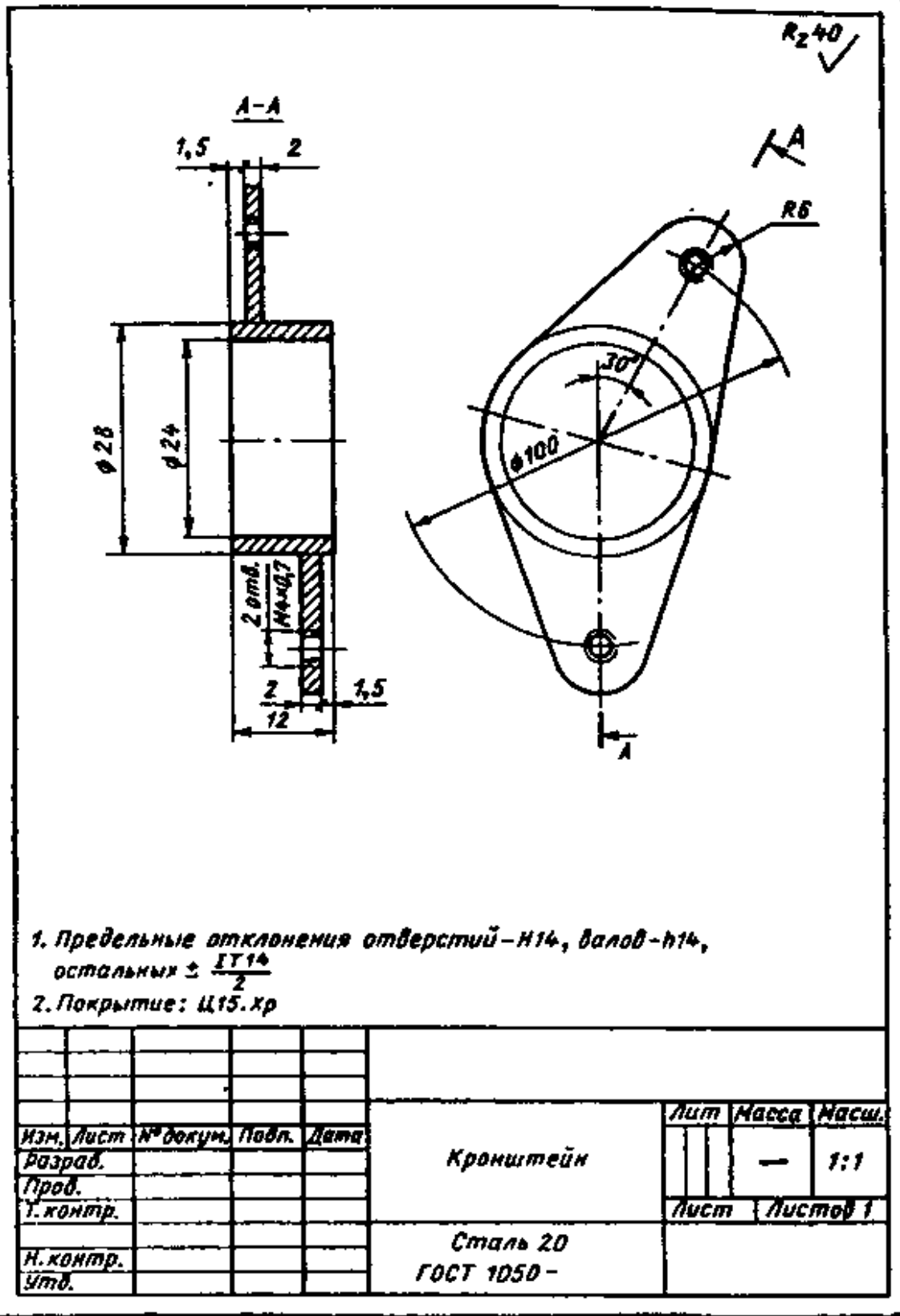
Рисунок 4- Пример оформления чертежа детали, формат А4
