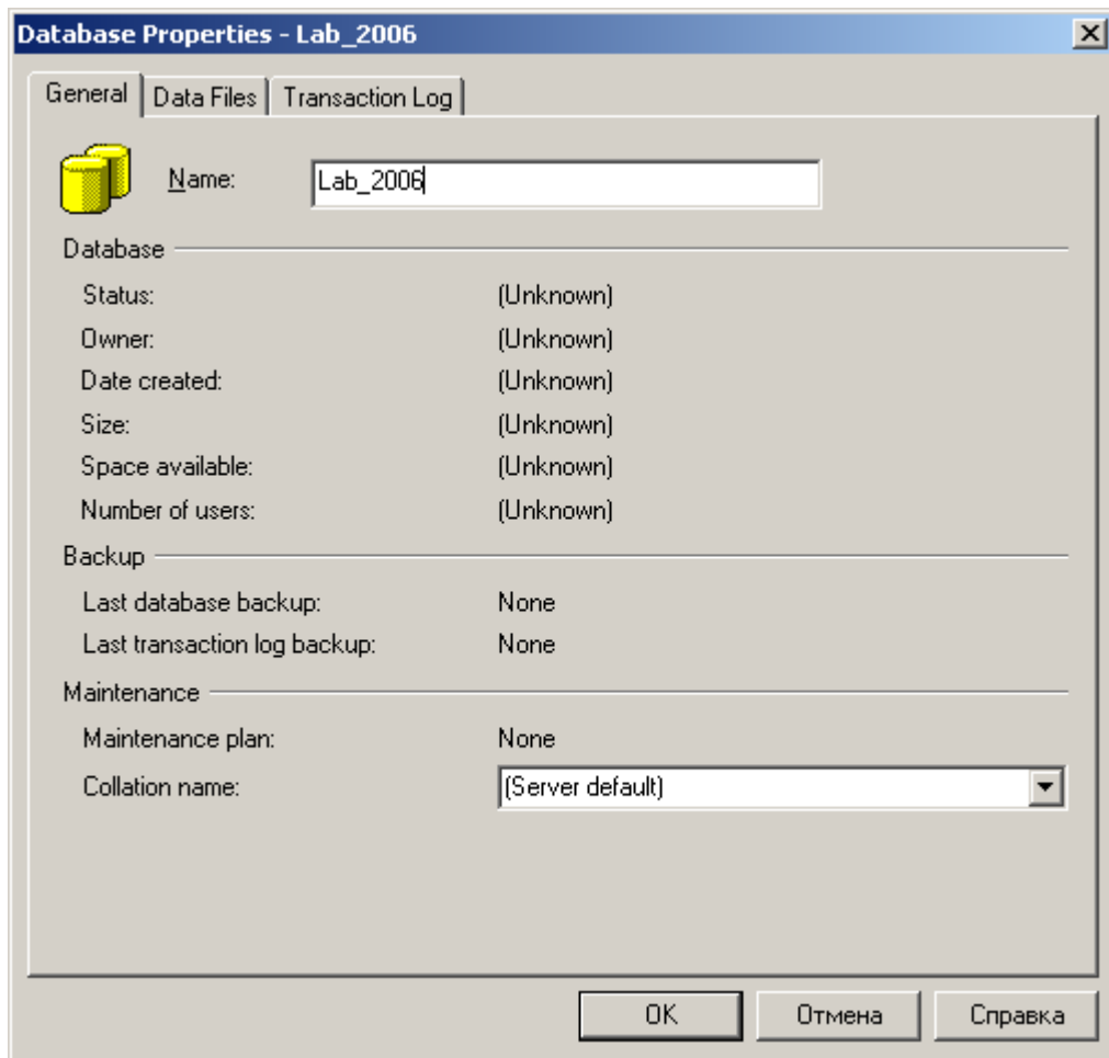
Рис 3.2. Вкладка General
