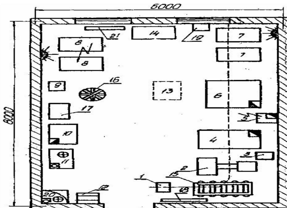
Экспликация оборудования
