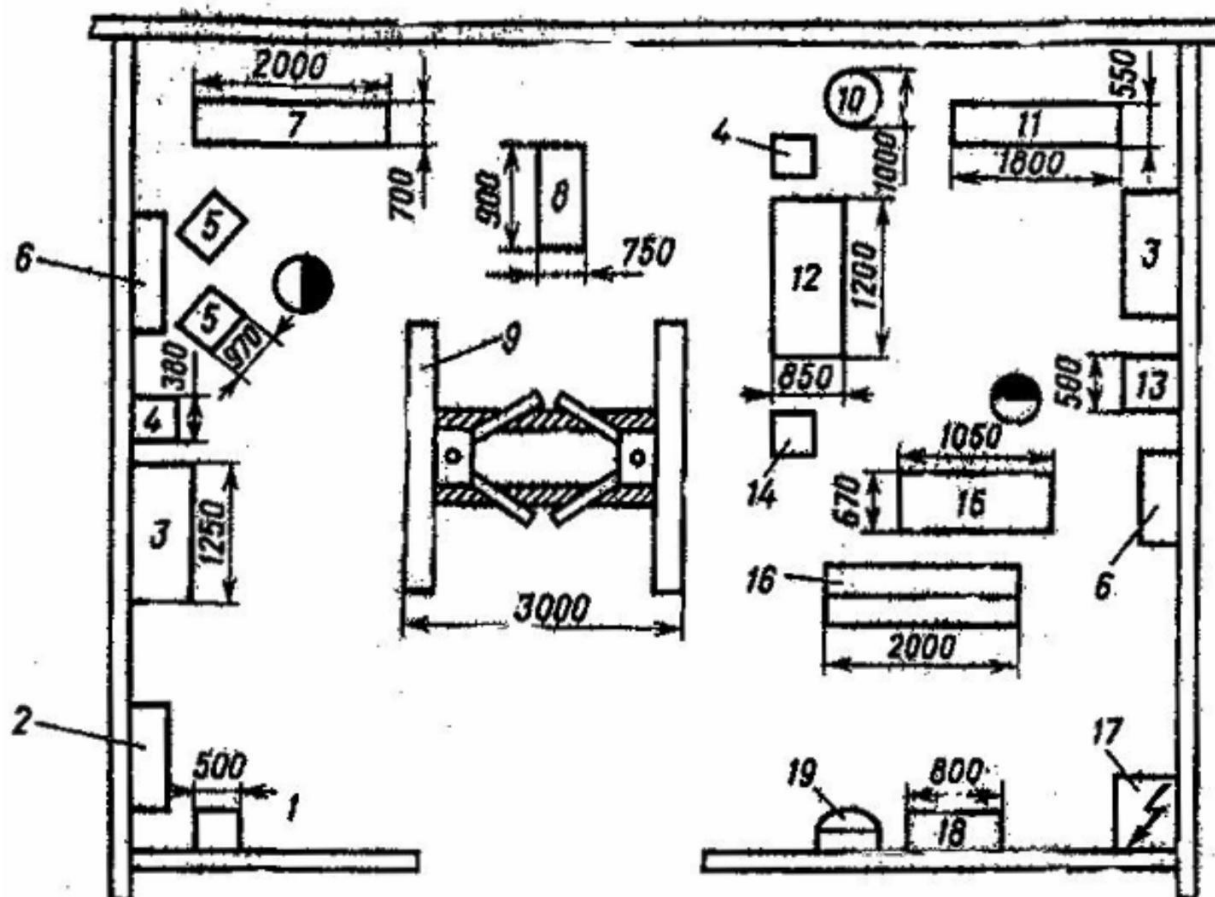
Экспликация оборудования
