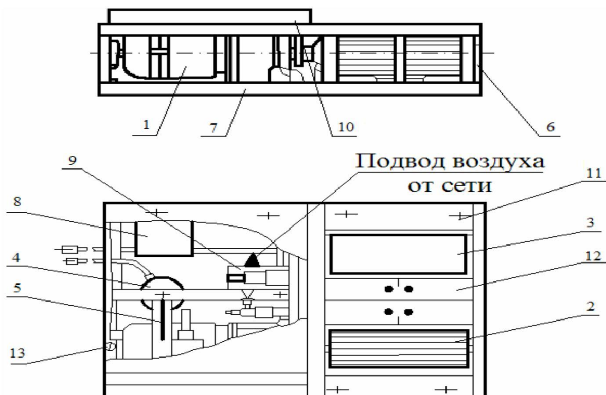
Рисунок 6 - Блоки роликов: 1 – мотор-редуктор; 2 – ведущий ролик; 3 – поддерживающий ролик; 4 – датчик силоизмерительной системы; 5 – рычаг; 6 – опоры; 7 – рама; 8 – коробка; 9 – пневмораспределитель; 10 – крышка; 11 – трап; 12 – подъемник; 13 – болт заземления
